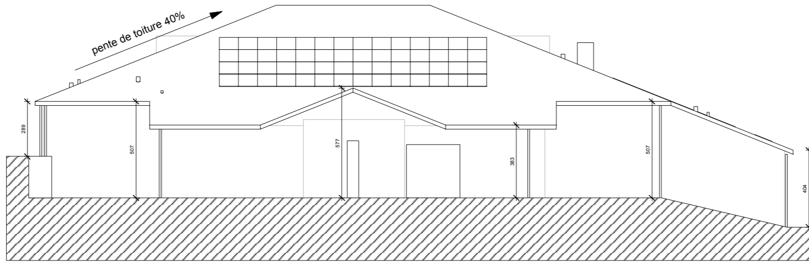
FACADE SUD OUEST
